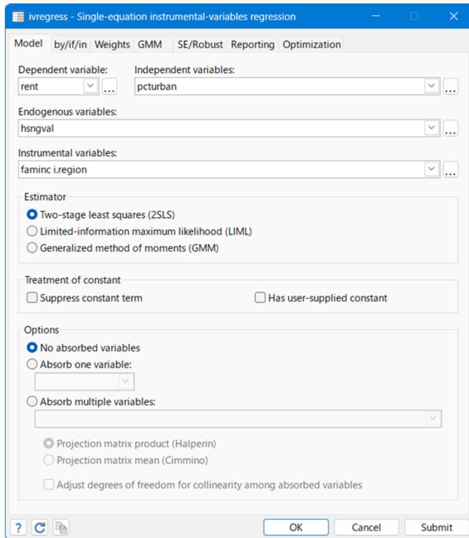
図 1 ivregress ダイアログ - Model タブ
